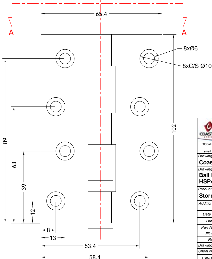
Section A-A
