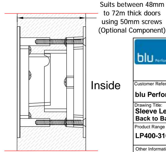
Section D-D
