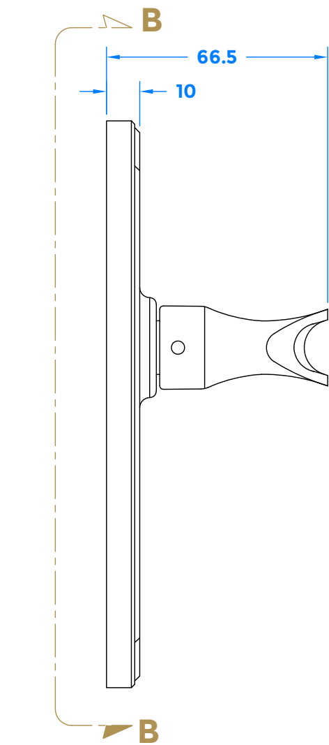
Section A-A
