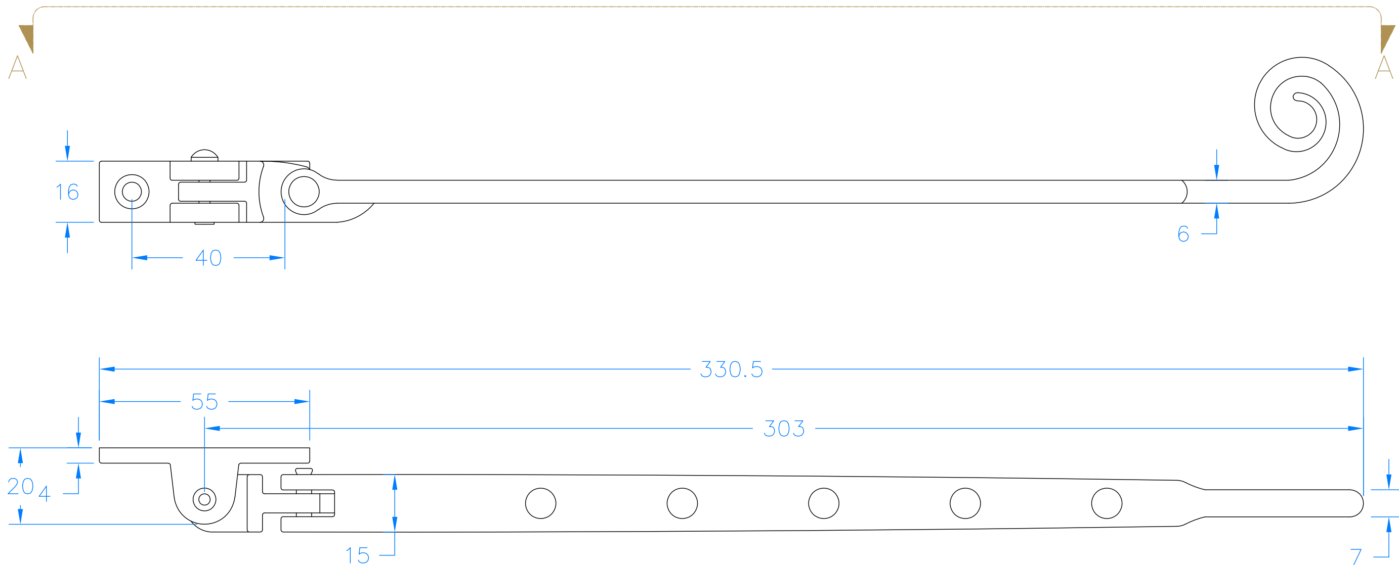
Section A-A
