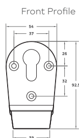
Internal Escutcheon
