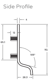
External Escutcheon
