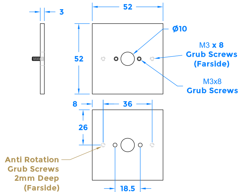
External Mounting Plate (Pull Side Shown)
