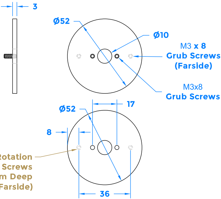
External Mounting Plate (Pull Side Shown)
