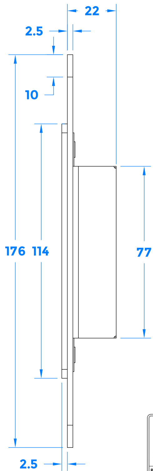
Section A-A
