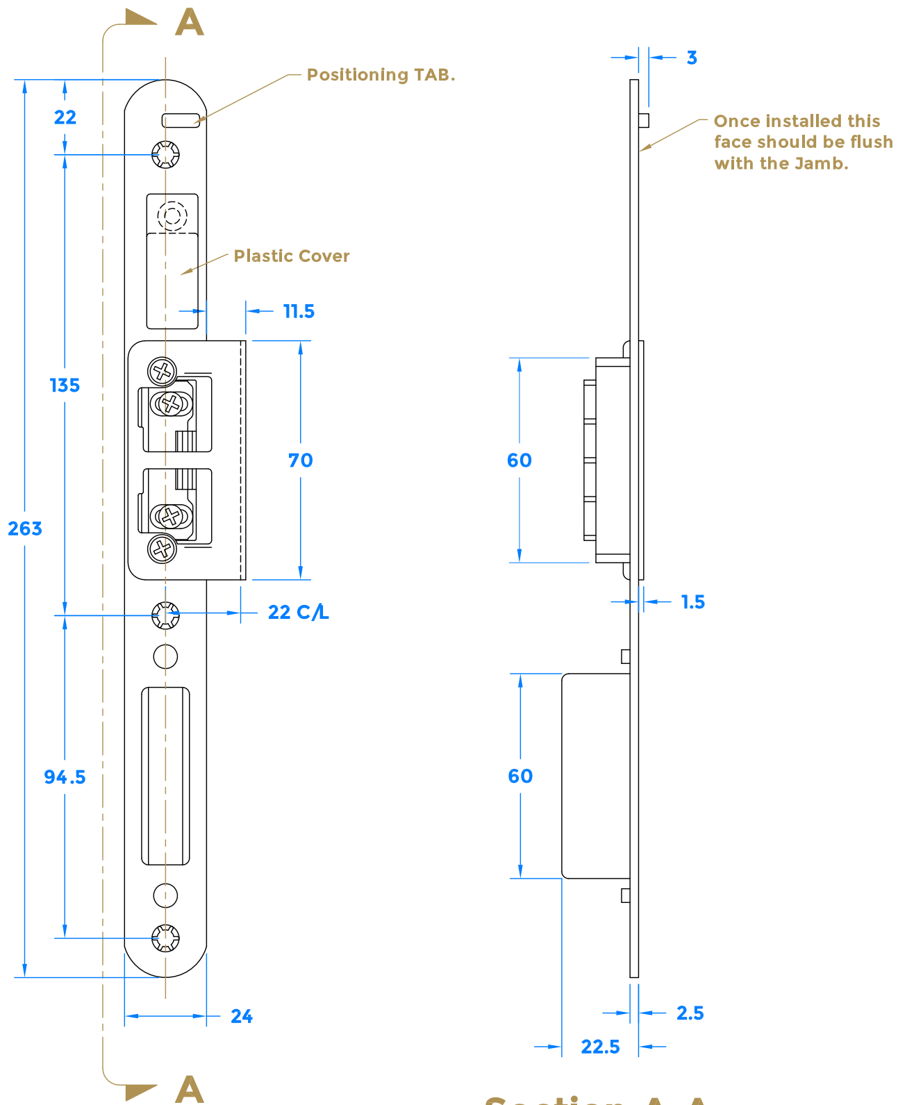
Section A-A
