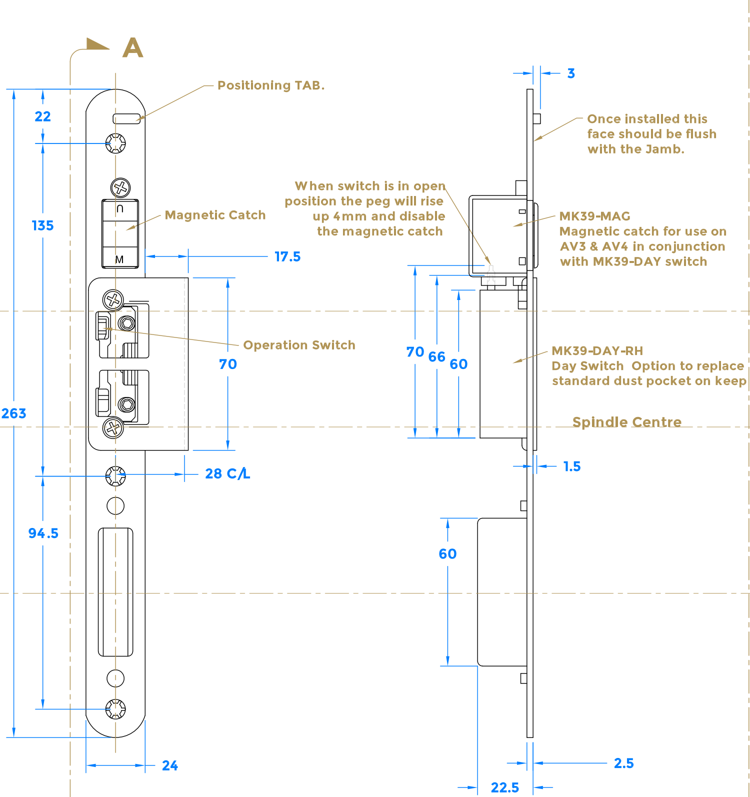
Section A-A
