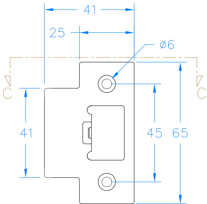
Striker
