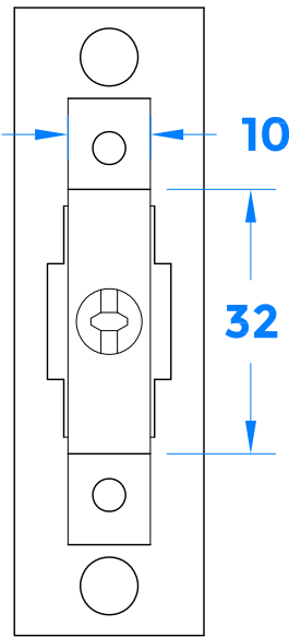
Section D-D
