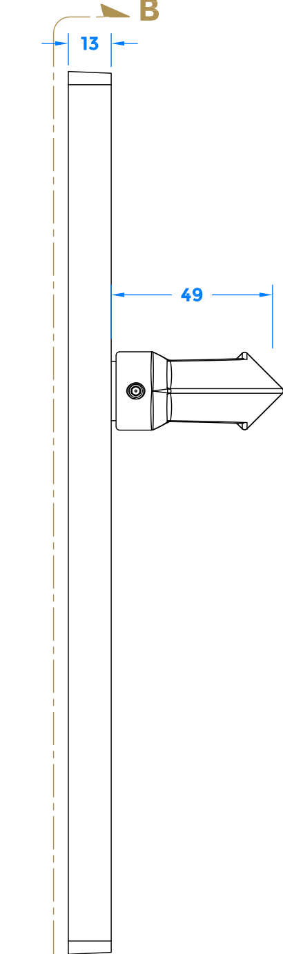
Section A-A
