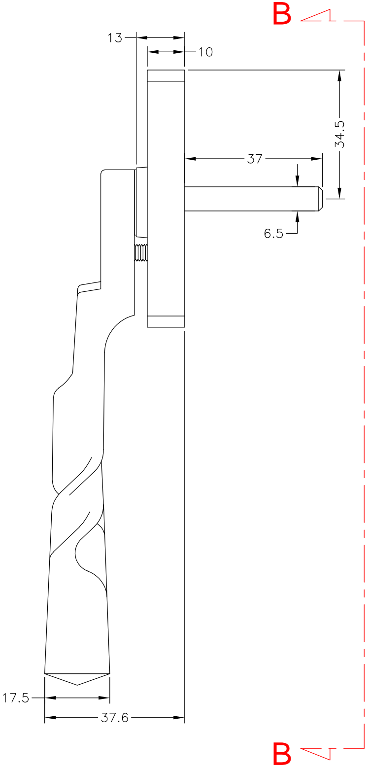
Section A-A
