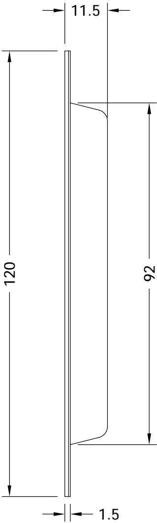
Section A-A
