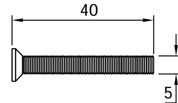
M5 x 40 BOLT
