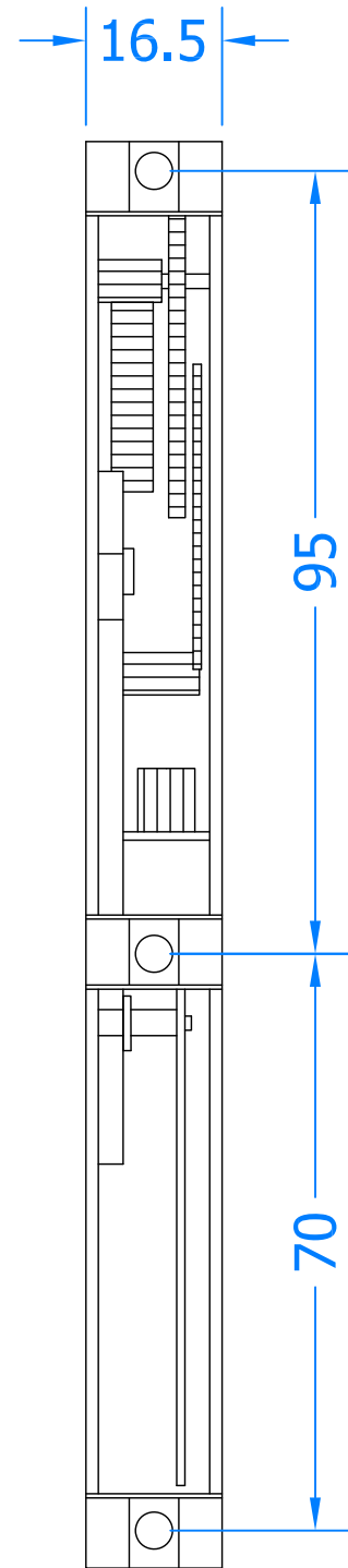
Section A-A
