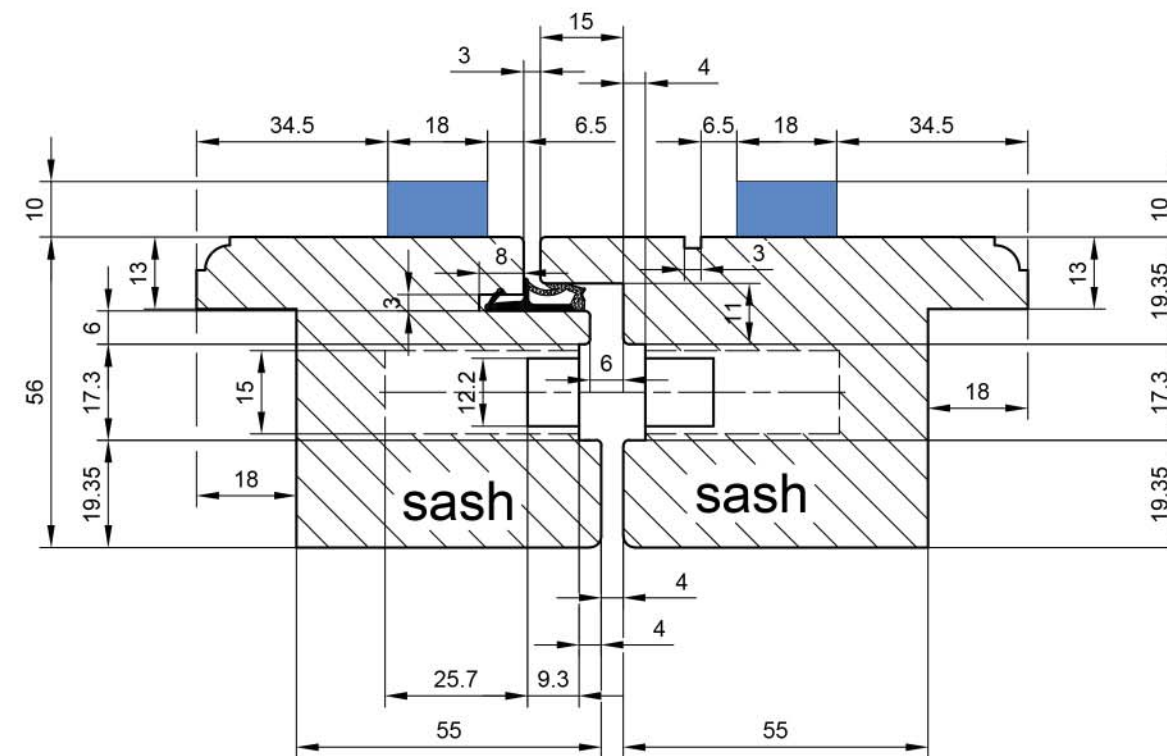
Lock edge detail
