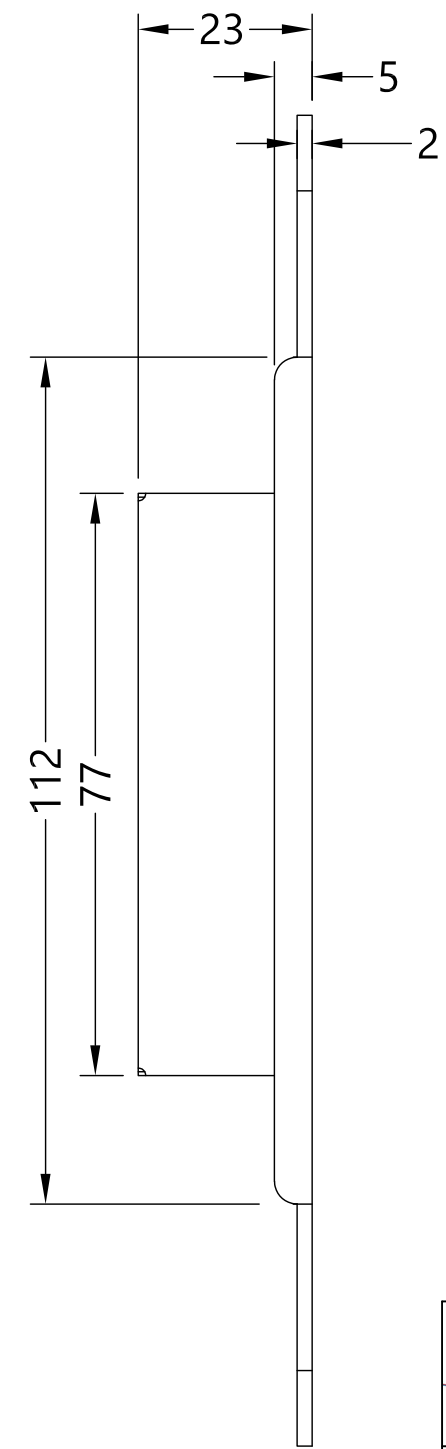
Section A-A
