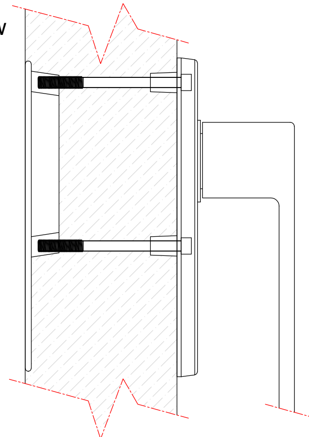
Section A-A
