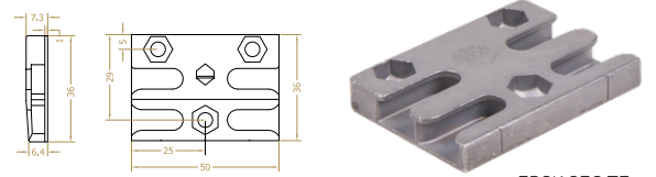
EBSK-SEC-TE
