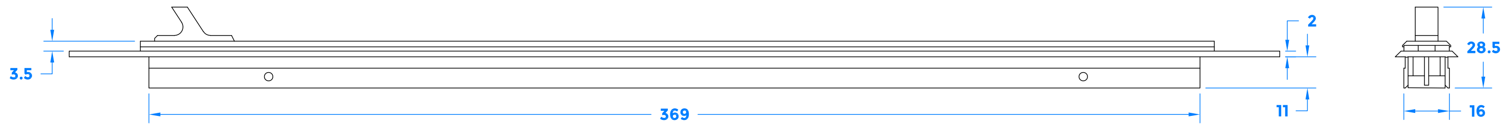
Section A-A
